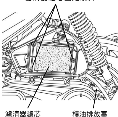
濾清器濾芯固定螺絲
