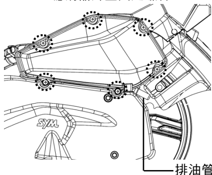
濾清器外蓋固定螺絲
