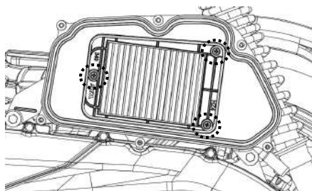
濾清器濾芯固定螺絲
