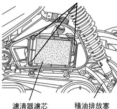
濾清器濾芯 固定螺絲
