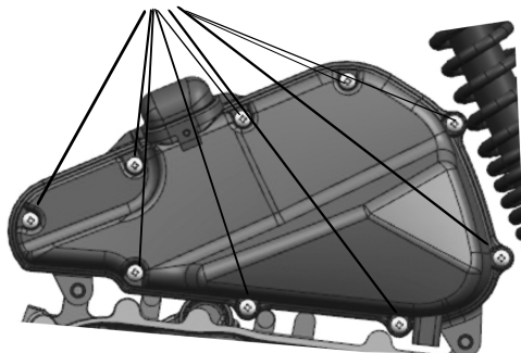
濾清器蓋固定螺絲
