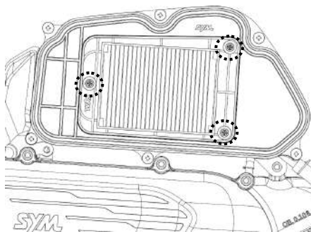
濾清器濾芯固定螺絲
