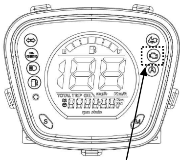
燃油噴射(EFI)故障警示燈
